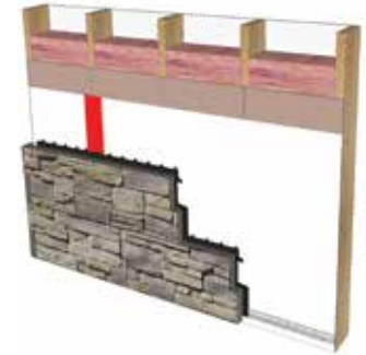
Charpente standard avec revêtement souple
