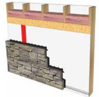
Charpente standard avec OSB ou contreplaqué et isolant rigide
